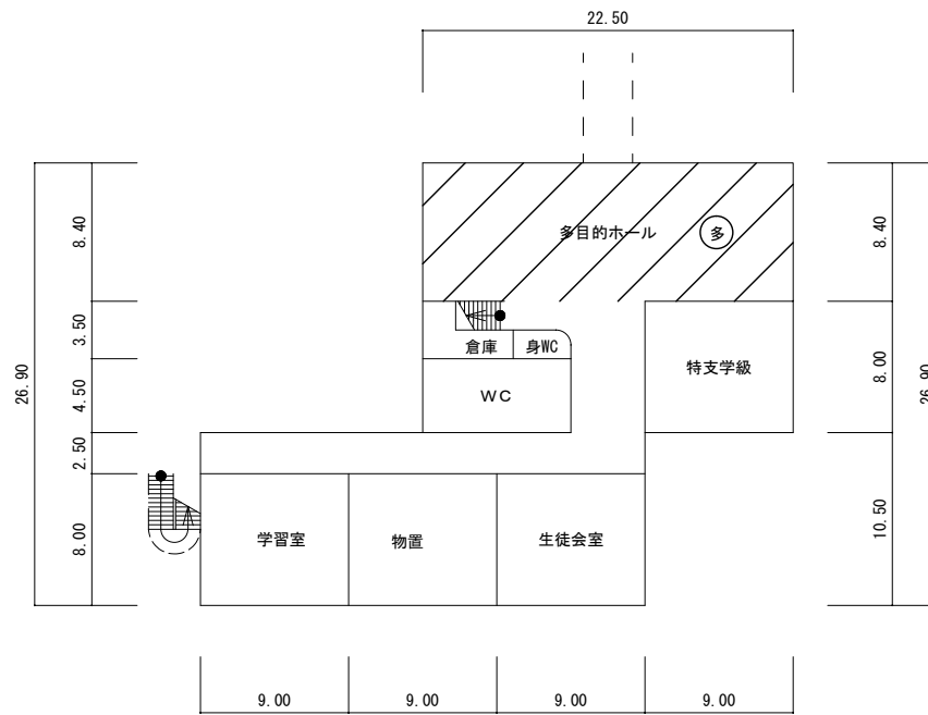
特別教室棟-1F
