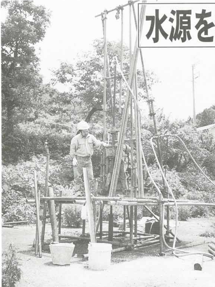
平成7年度から2年間にわたり町北部地域で行った水源調査（写真は杉生地内のボーリング調査）
