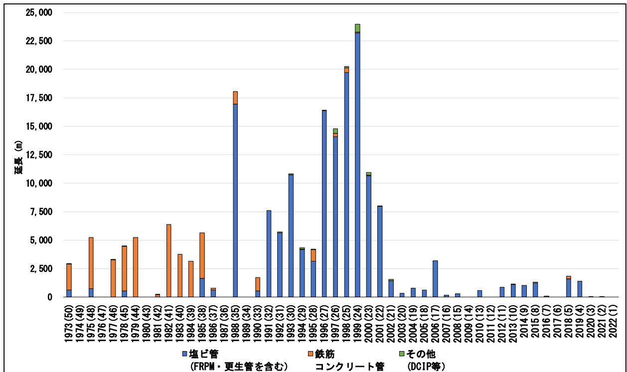
図 3-1 布設年度別管渠延長（污水管渠）
