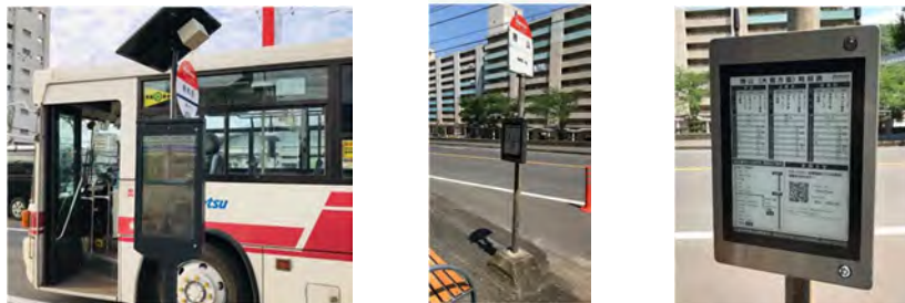
図 5.4 電源がない停留所での設置事例（西鉄バス）
